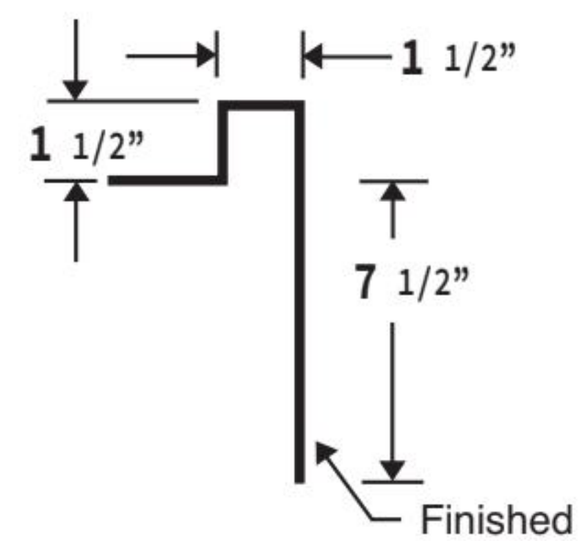
7" DOOR JAMB TRIM
