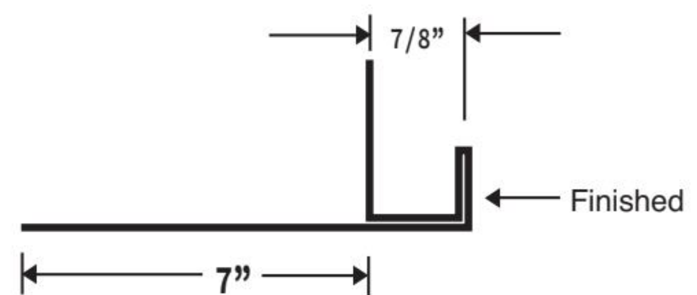
7" DOOR TRIM
