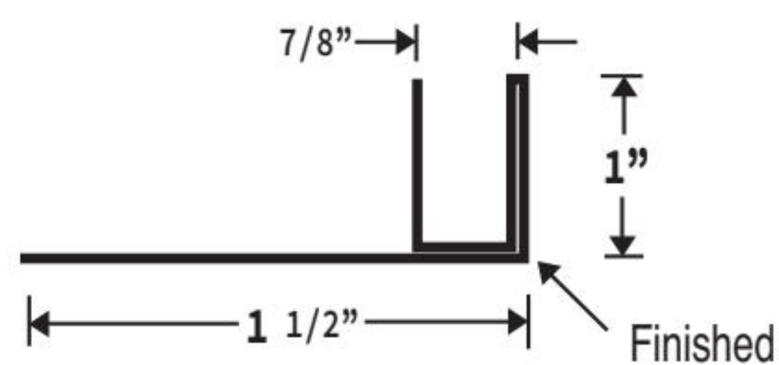
7/8" F TRIM
