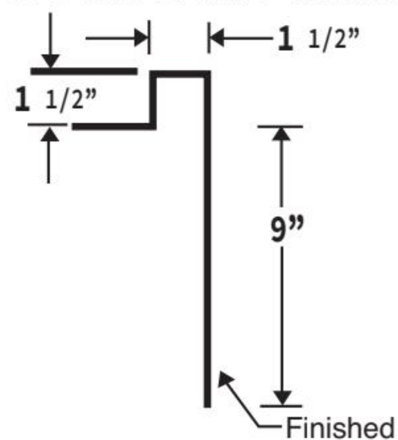
9" DOOR JAMB TRIM
