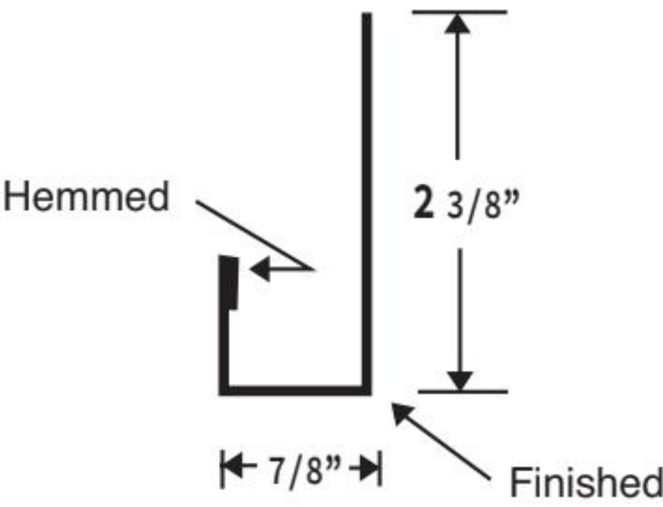
7/8" J TRIM
