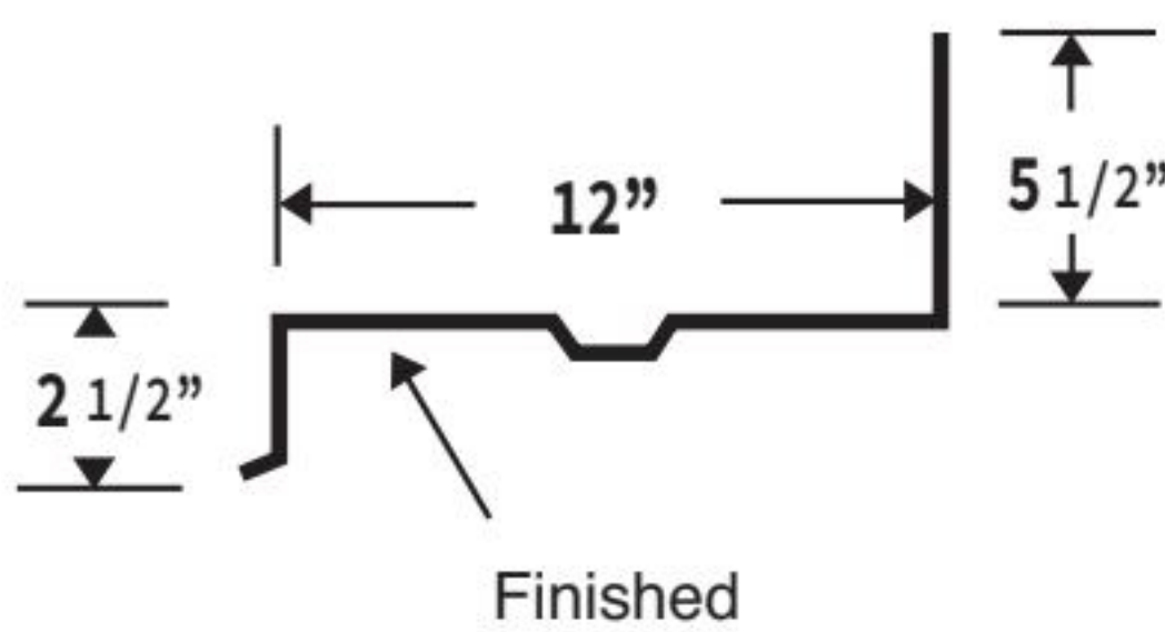
SOFFIT TRIM
