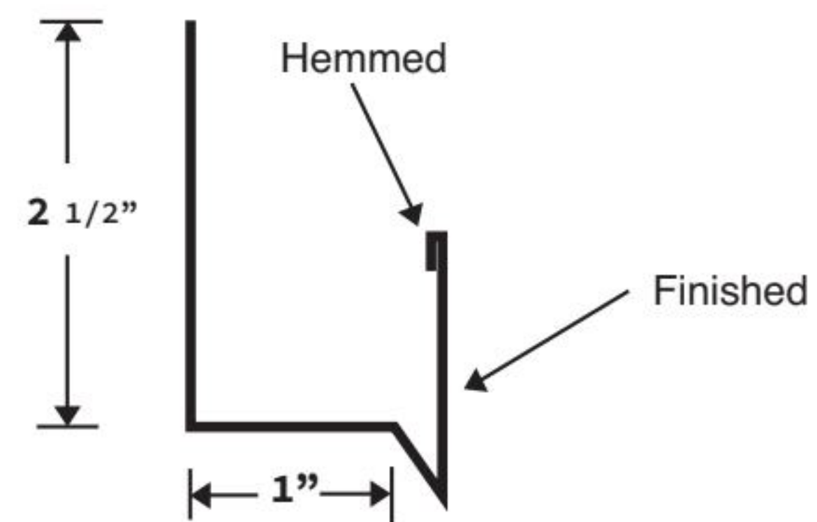
DOOR HEADER
