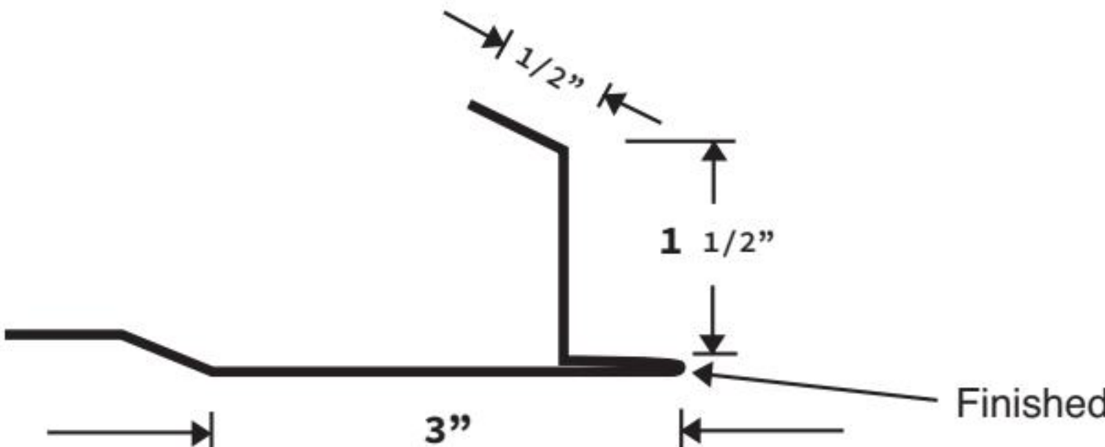
ASTRAGAL TRIM
