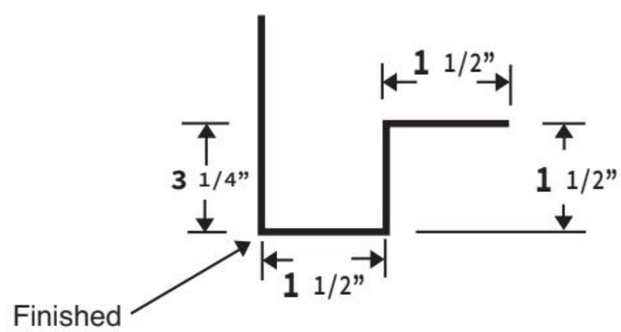
9" DOOR JAMB TRIM
